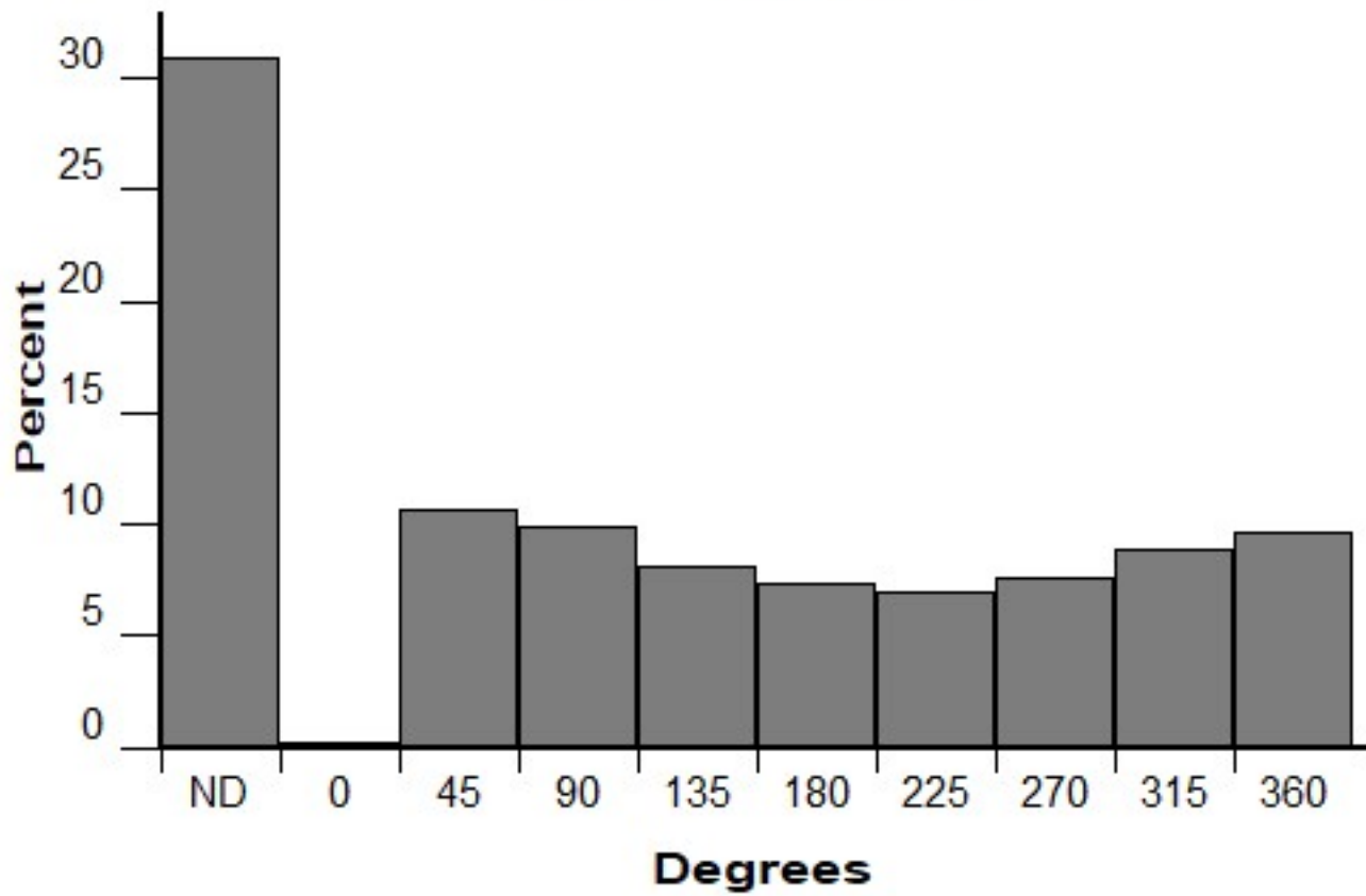
Aspect (FM 103)
