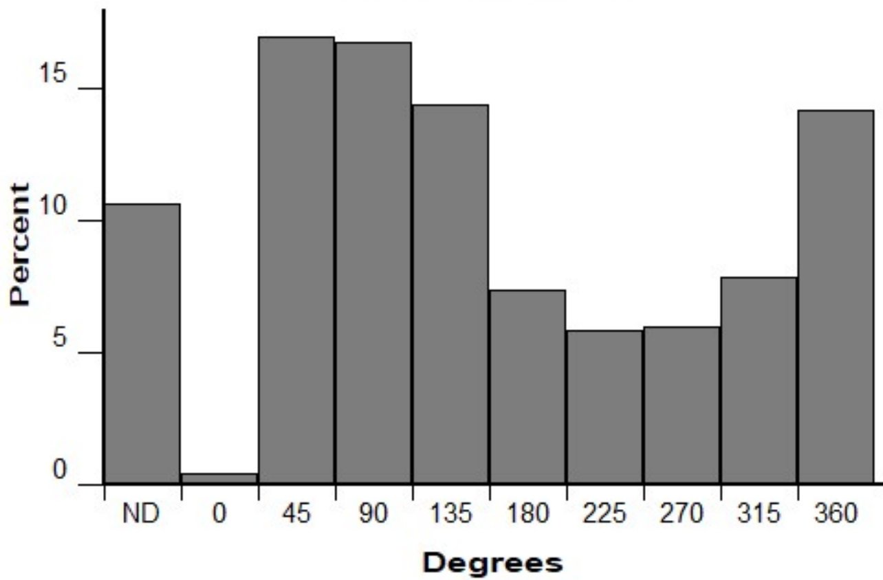
Aspect (FM 186)
