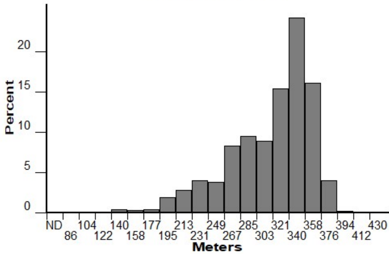
Elevation (FM 181)
