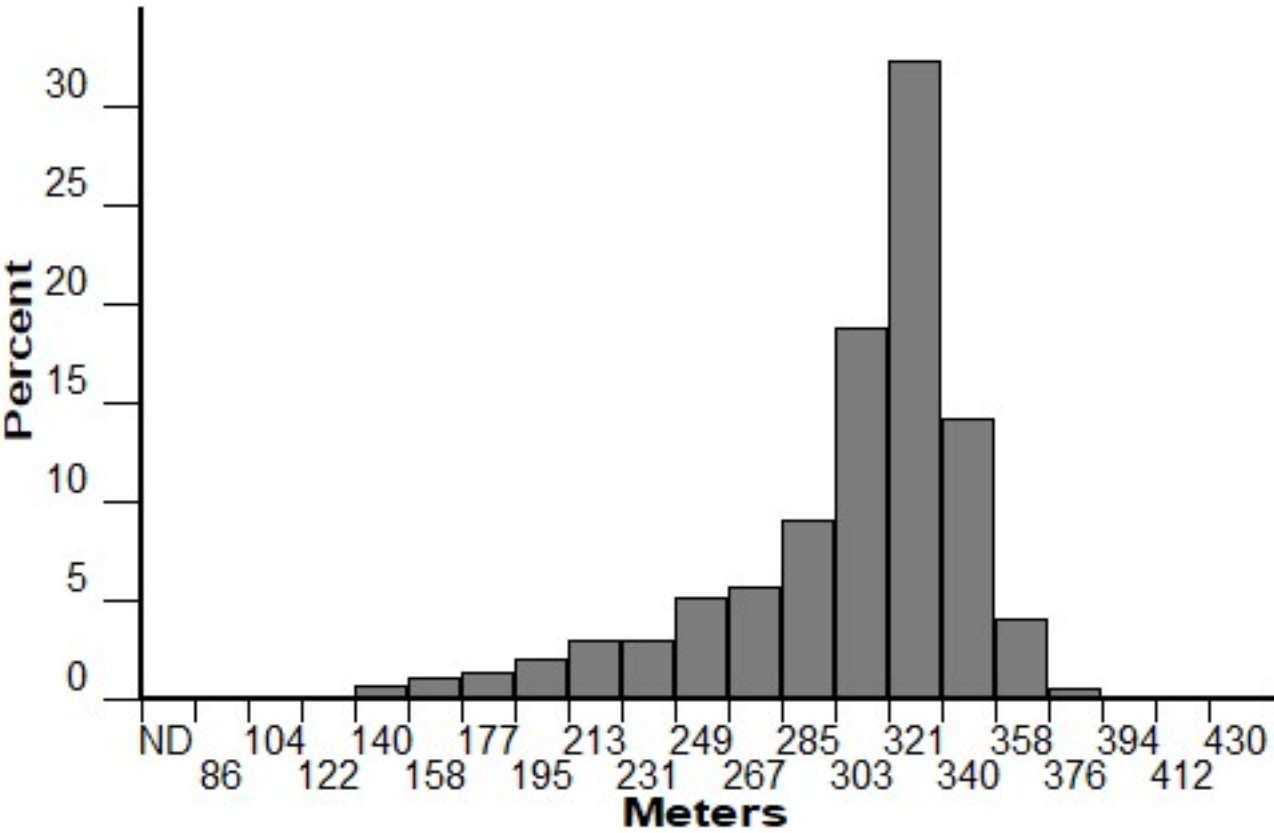
Elevation (FM 162)
