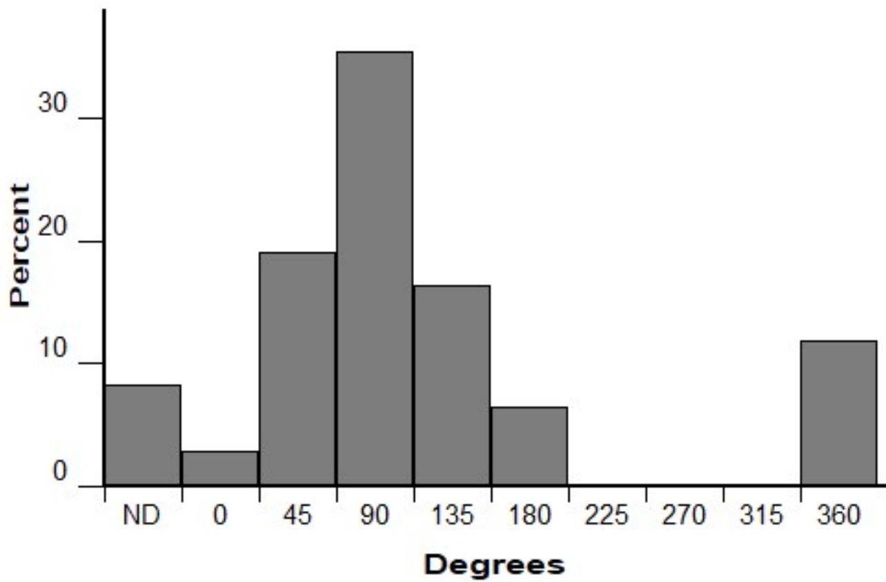
Aspect (FM 104)
