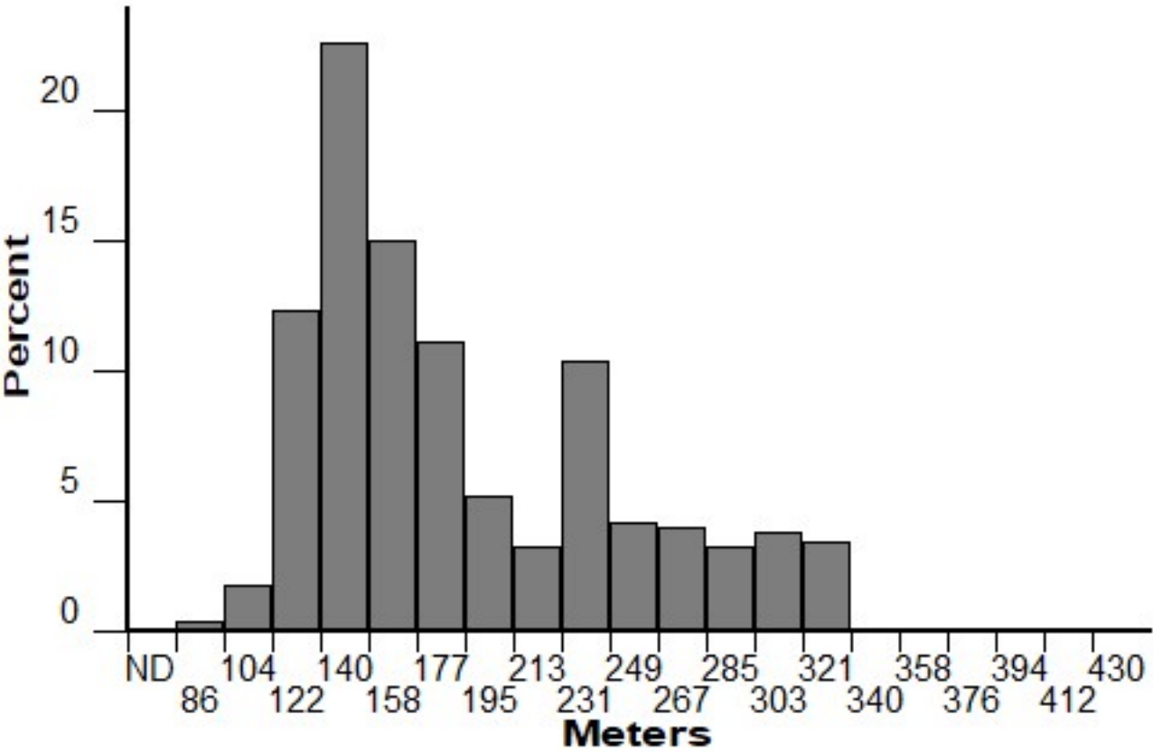
Elevation (FM 99)
