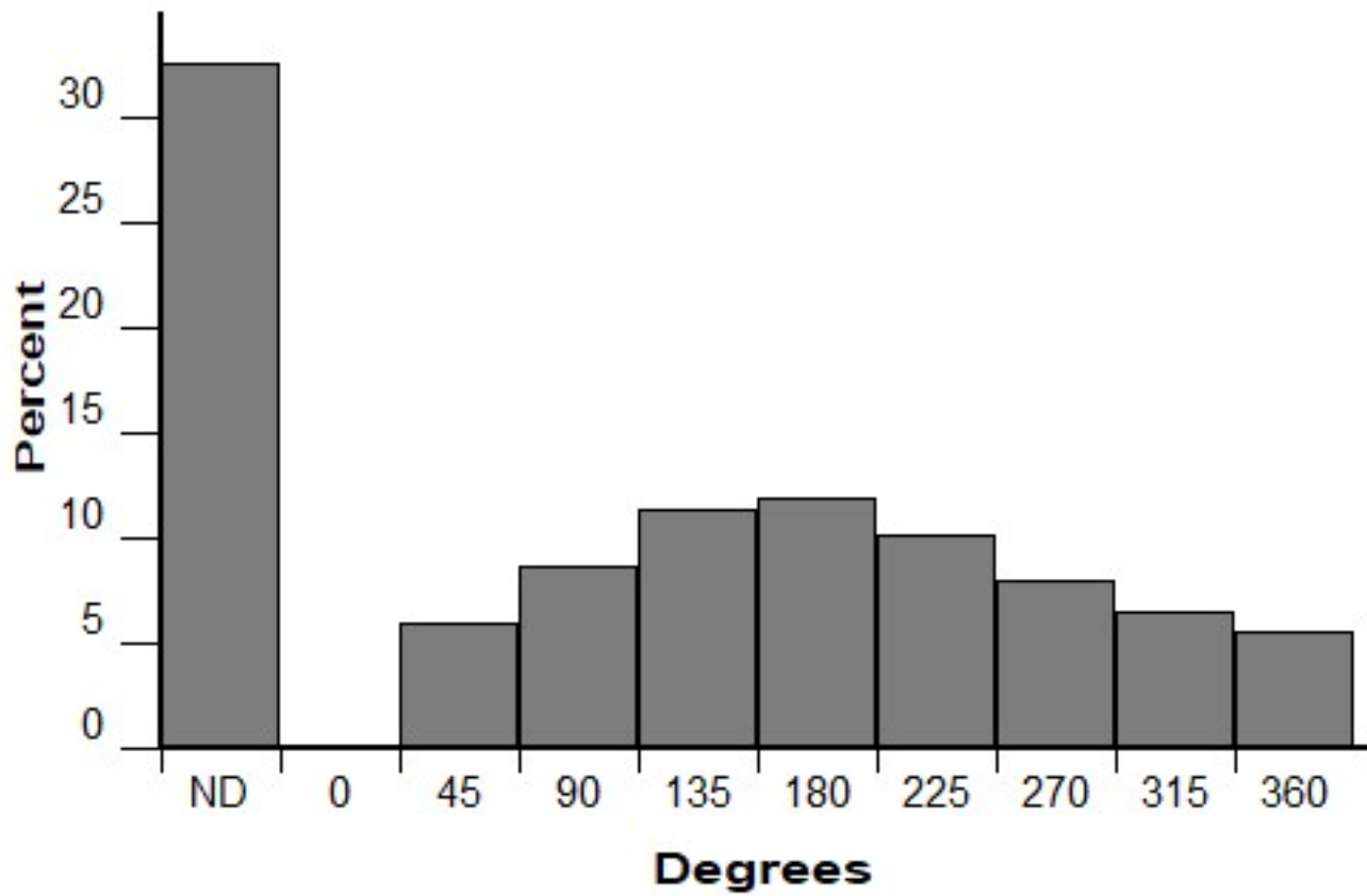
Aspect (FM 101)
