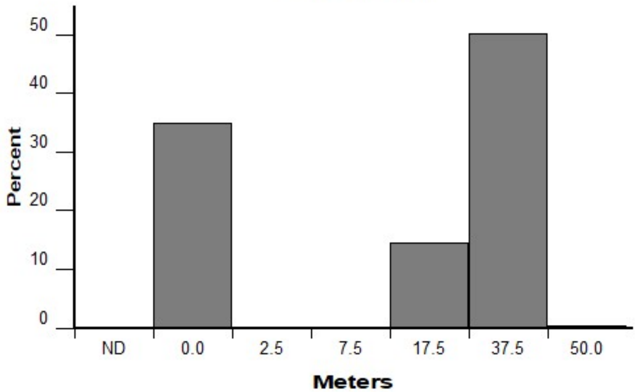
Stand Height
