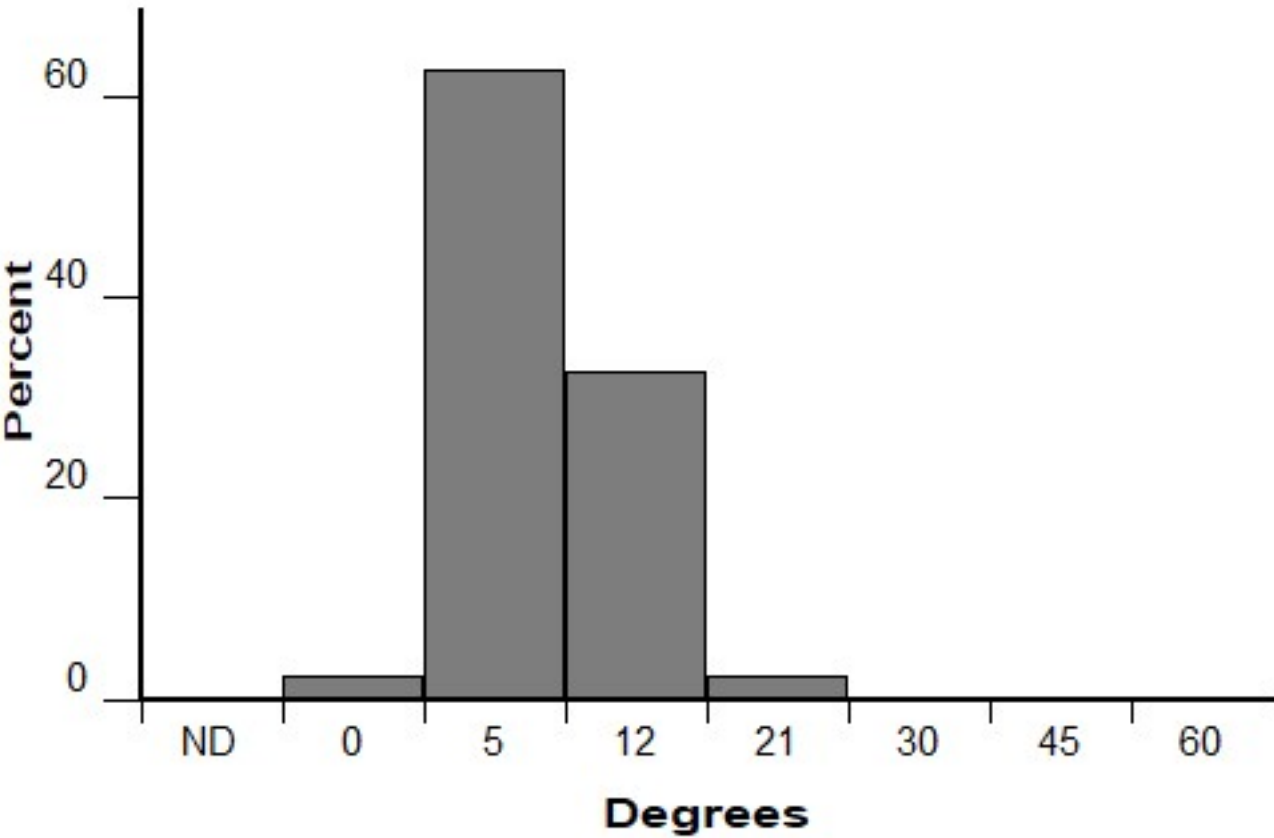
Slope (FM 146)
