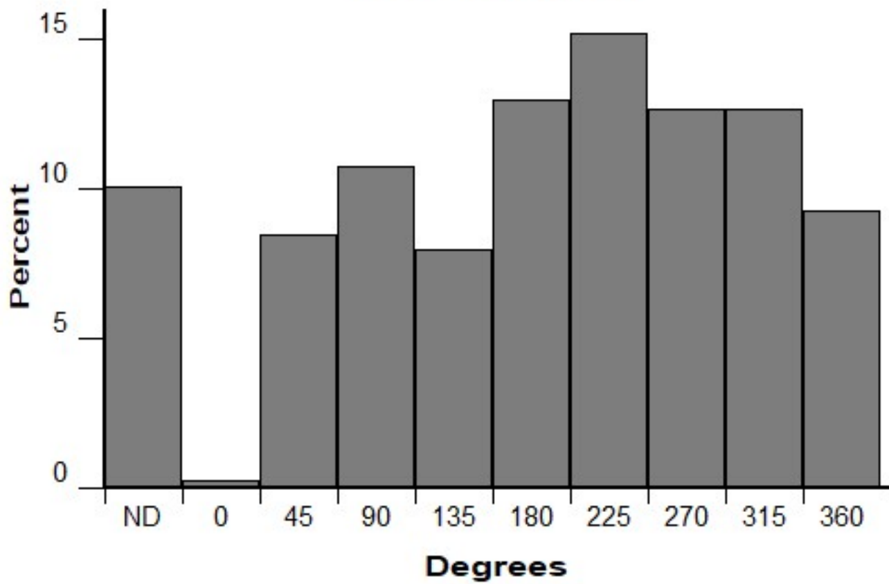
Aspect (FM 185)
