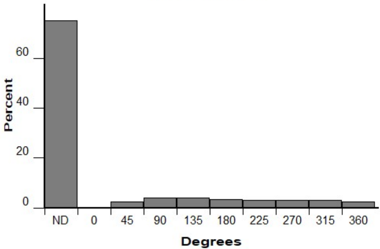
Aspect (FM 93)
