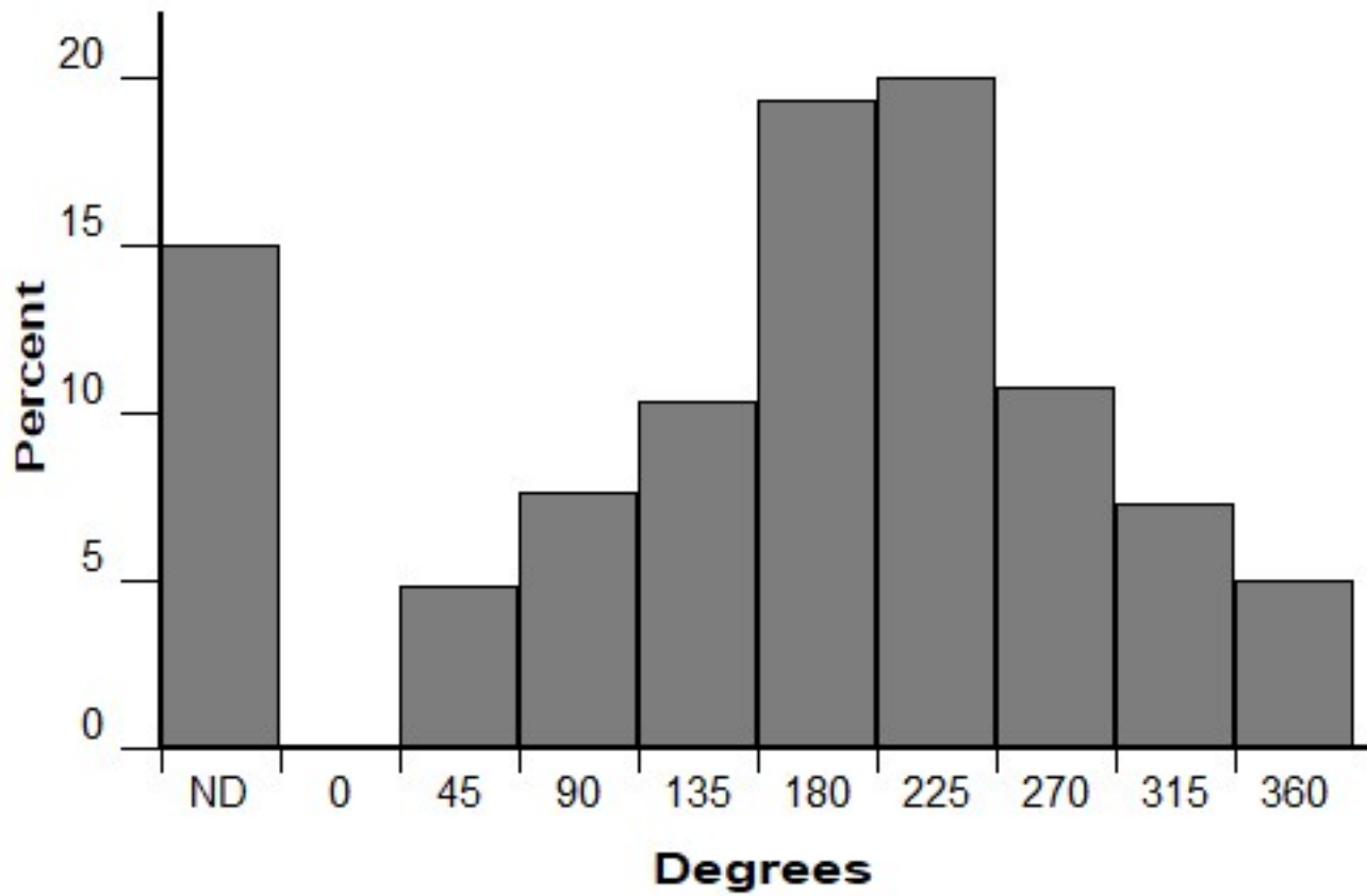
Aspect (FM 147)
