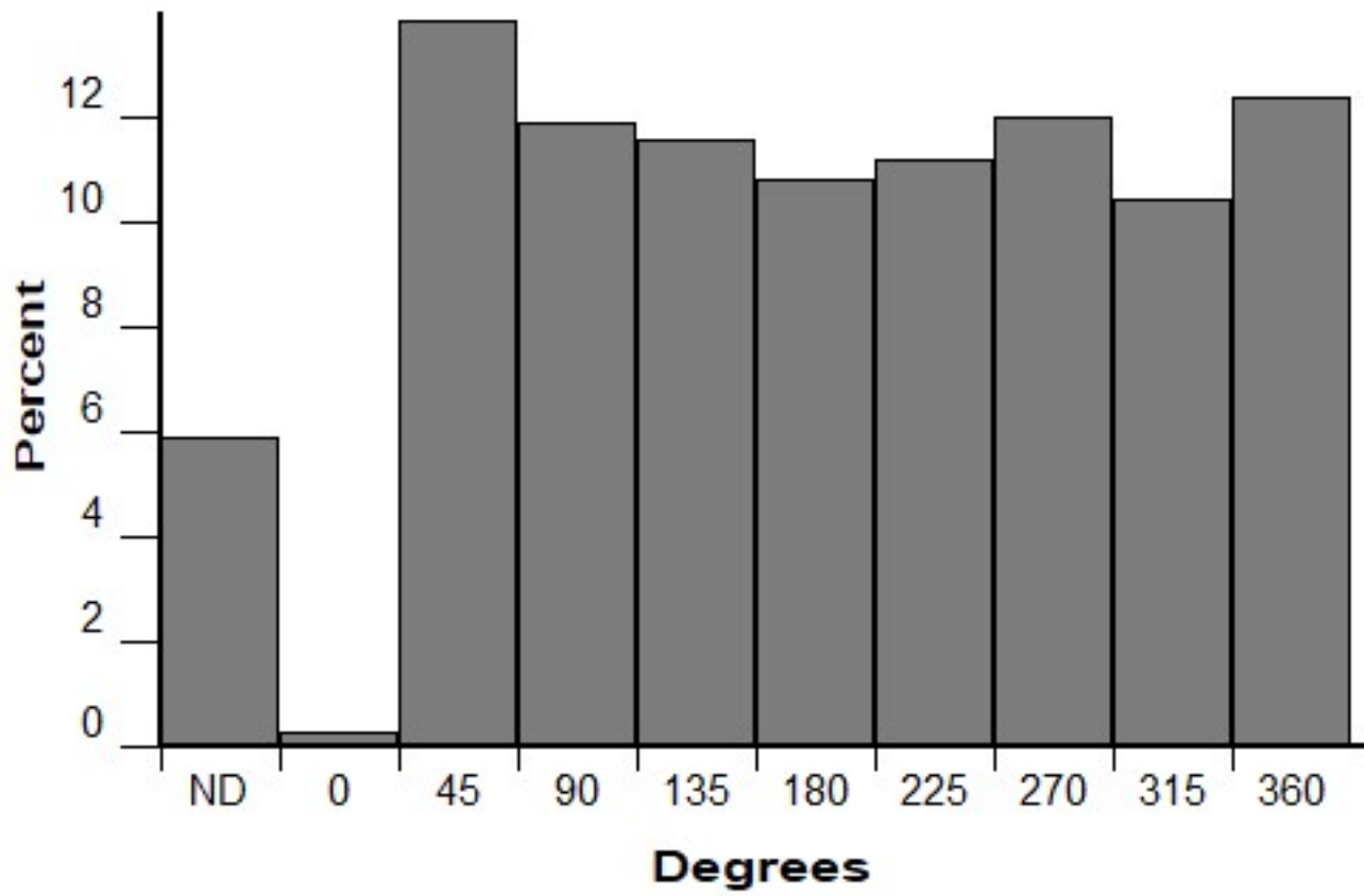
Aspect (FM 162)
