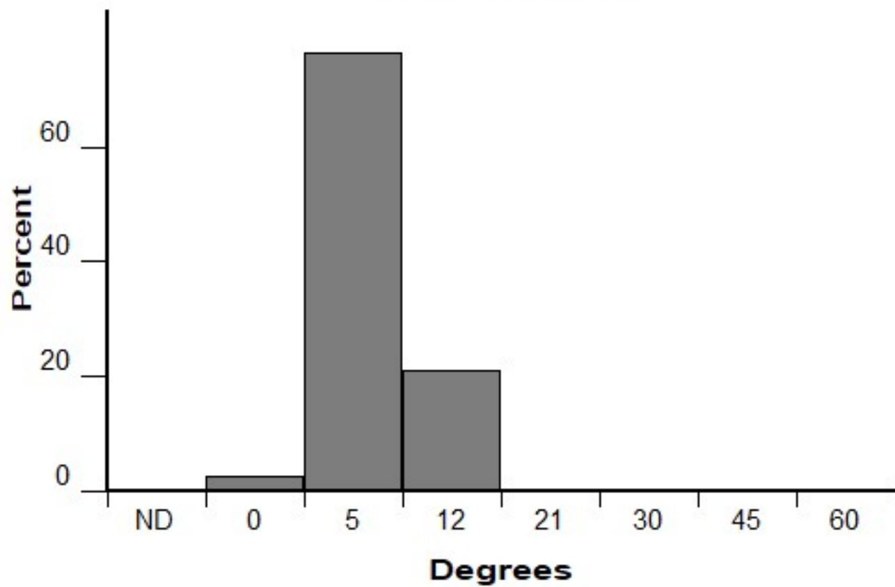
Slope (FM 144)
