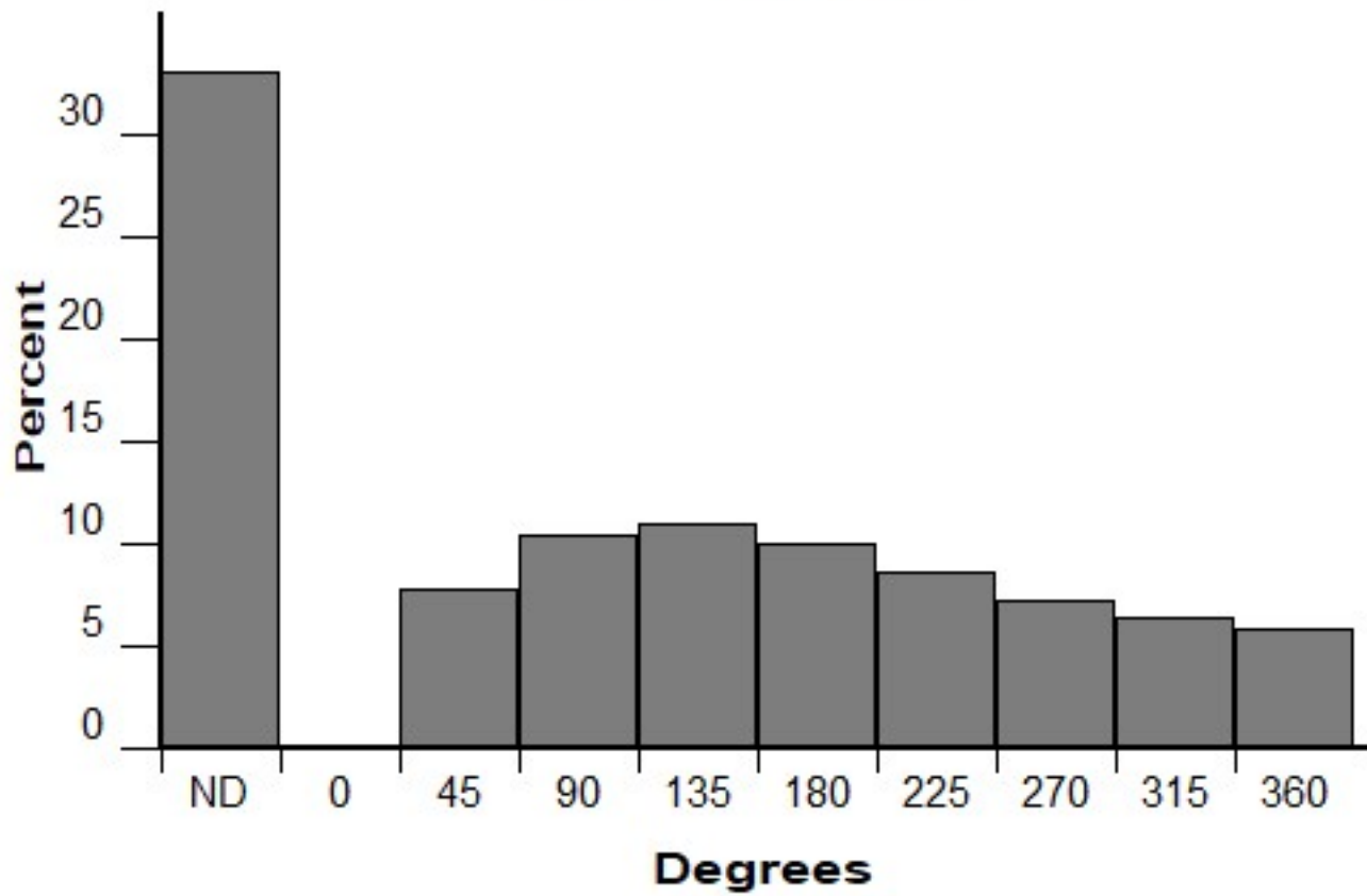
Aspect (FM 102)
