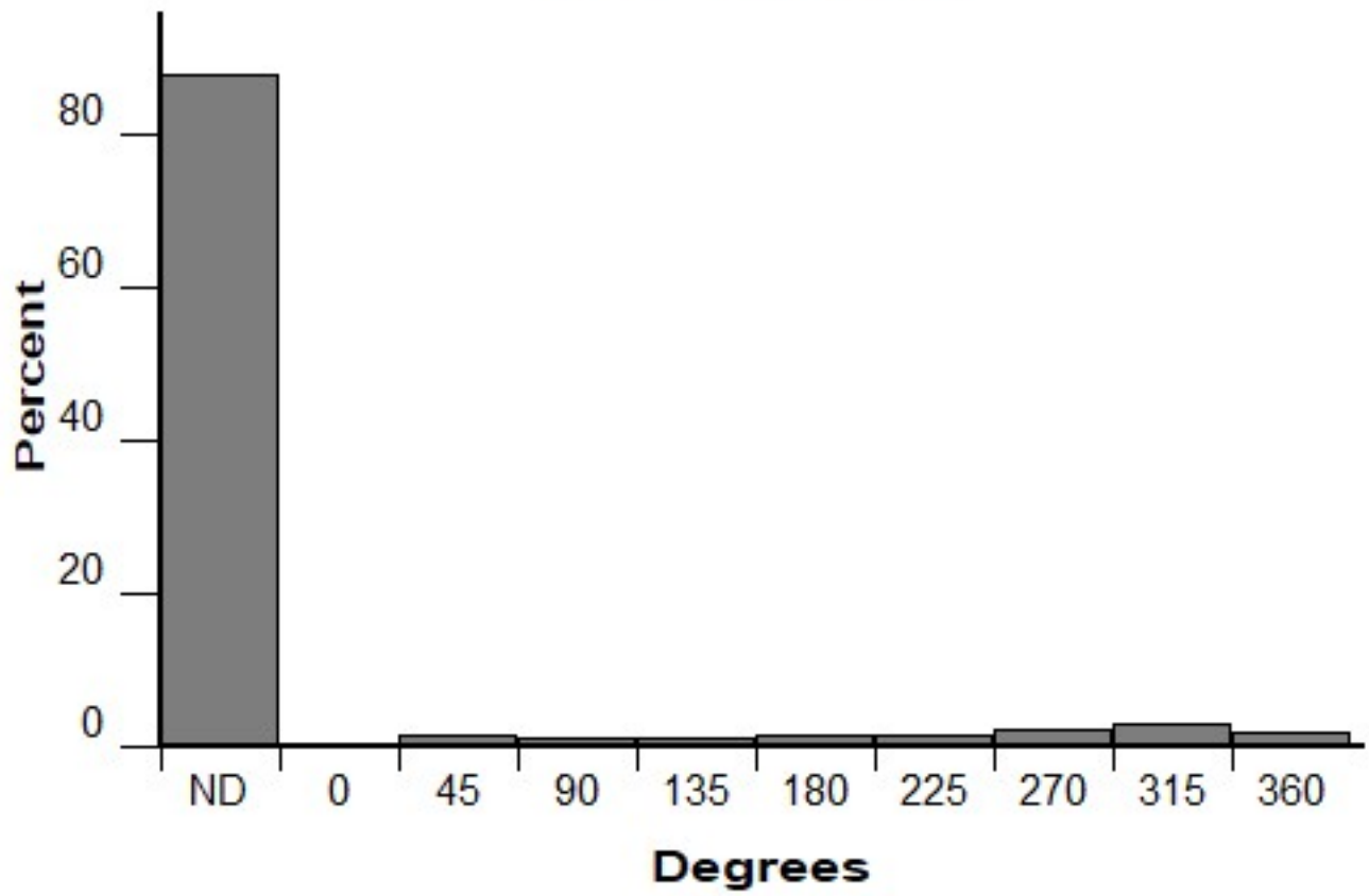
Aspect (FM 161)
