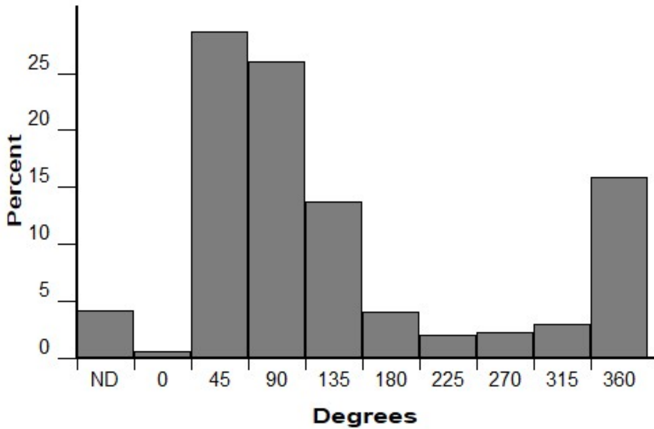
Aspect (FM 184)
