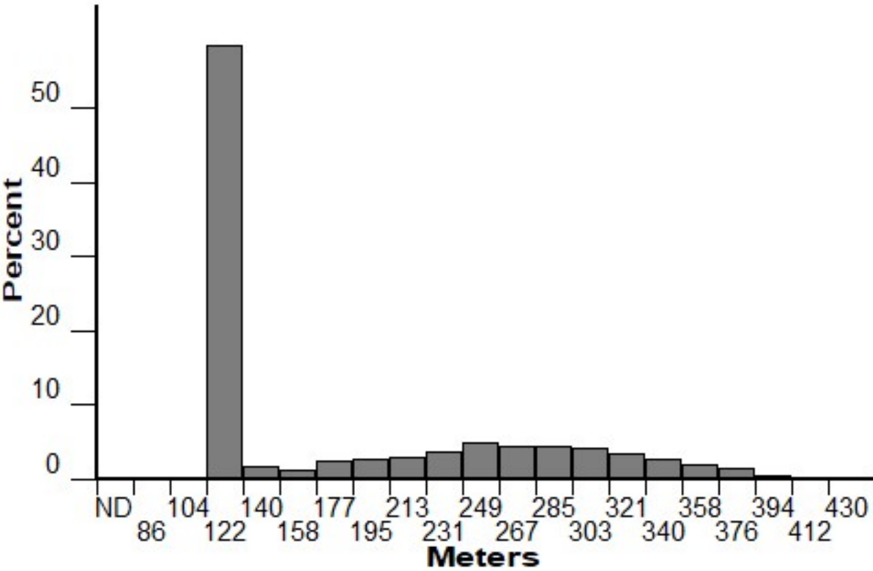
Elevation (FM 182)
