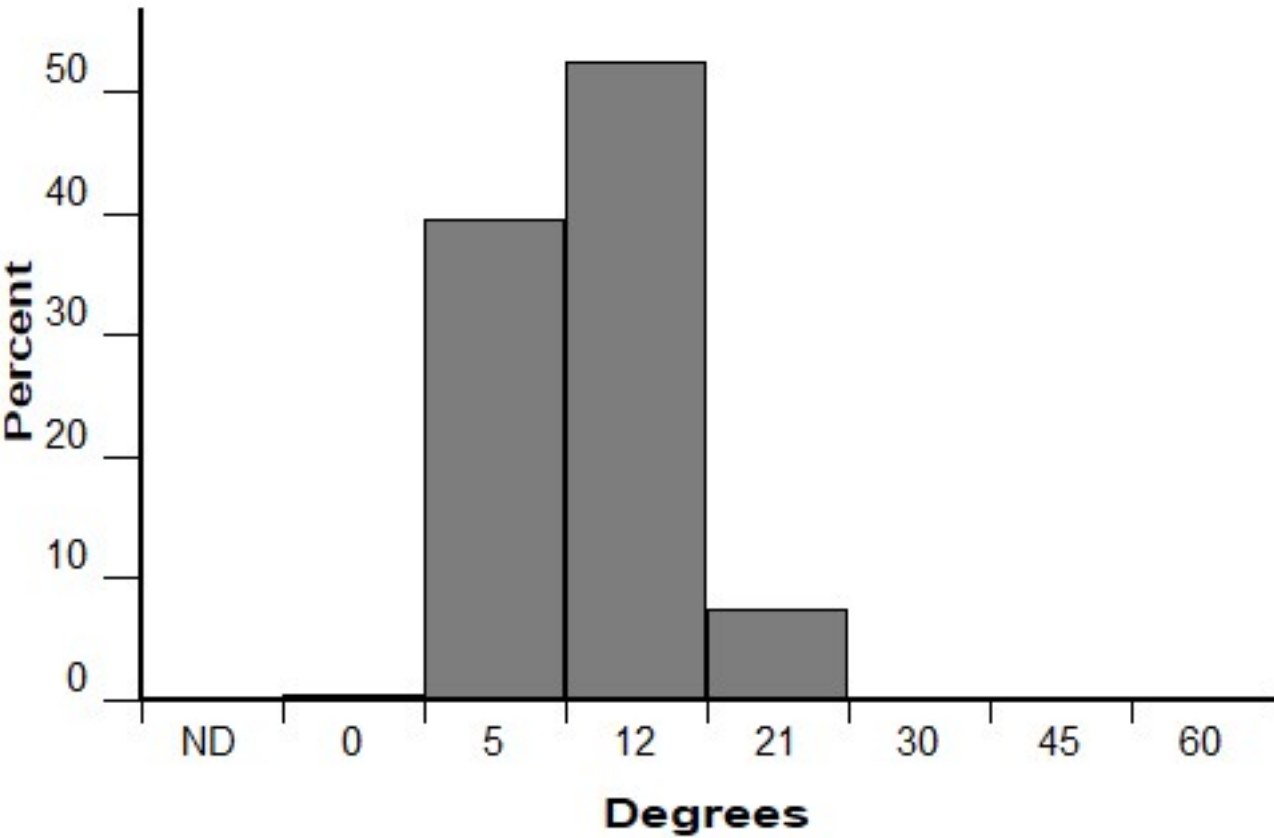
Slope (FM 185)
