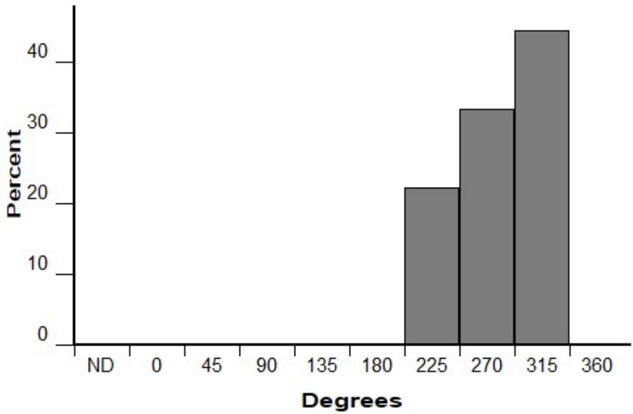
Aspect (FM 202)
