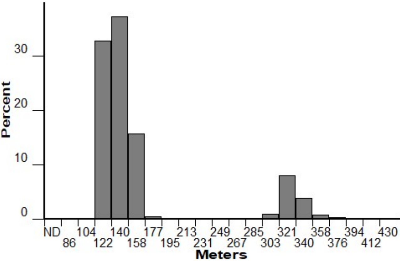
Elevation (FM 142)
