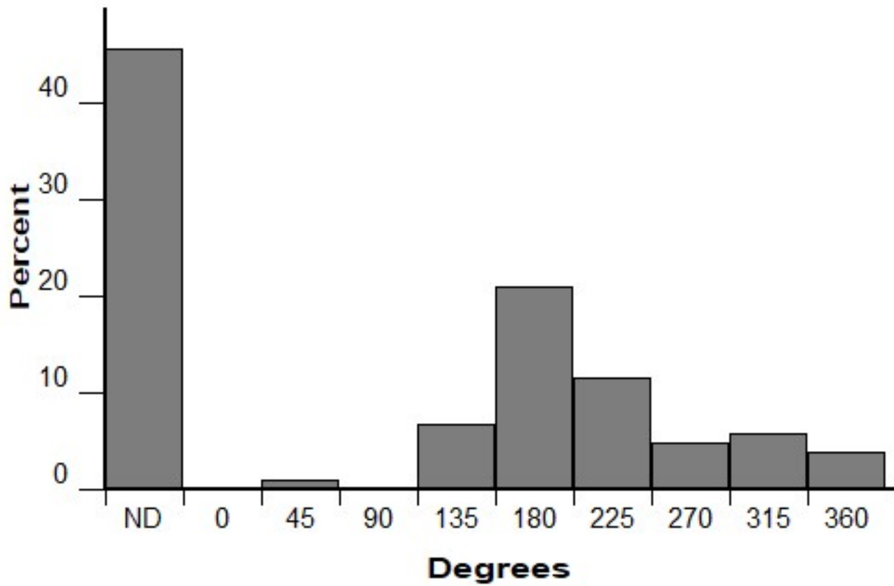
Aspect (FM 143)
