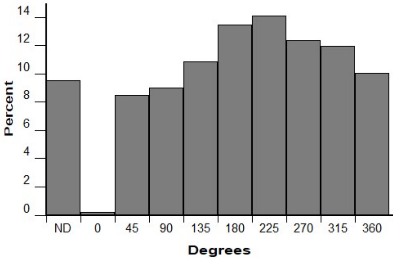
Aspect (FM 188)
