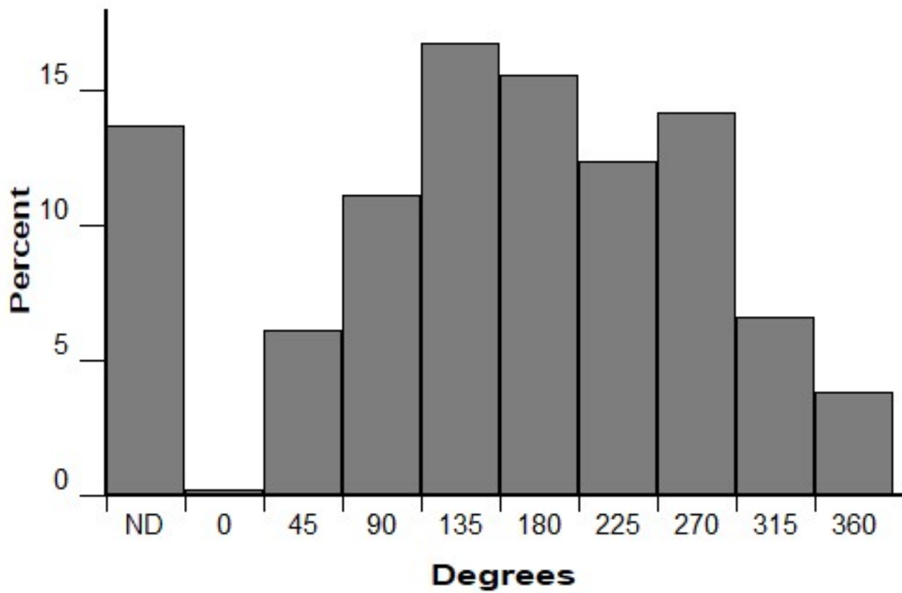
Aspect (FM 142)
