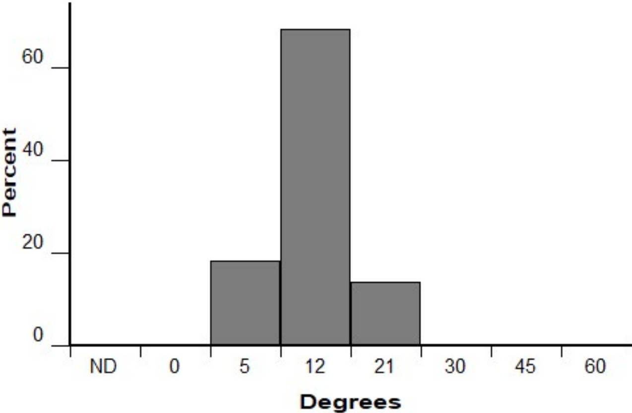
Slope (FM 184)
