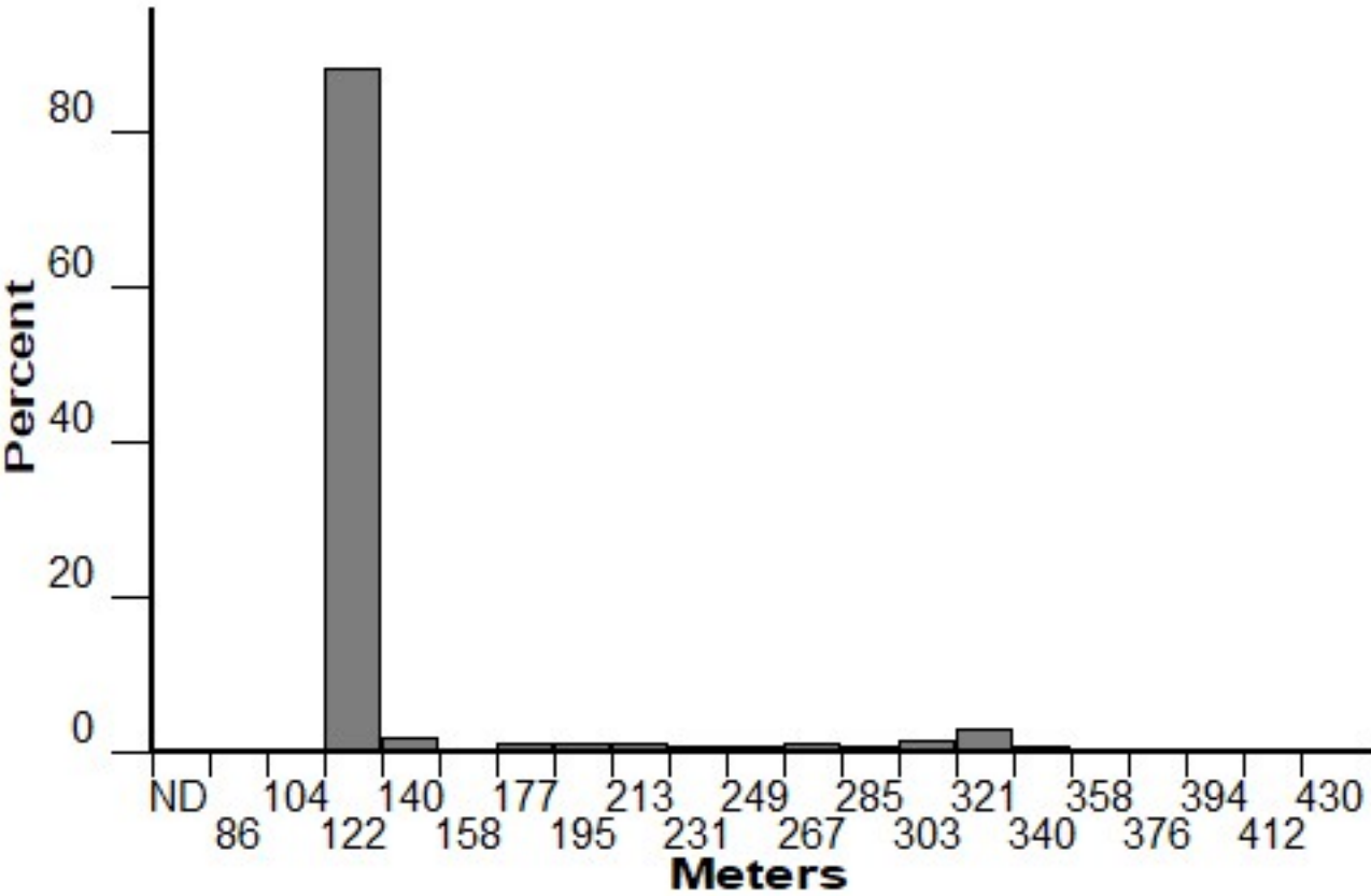
Elevation (FM 122)
