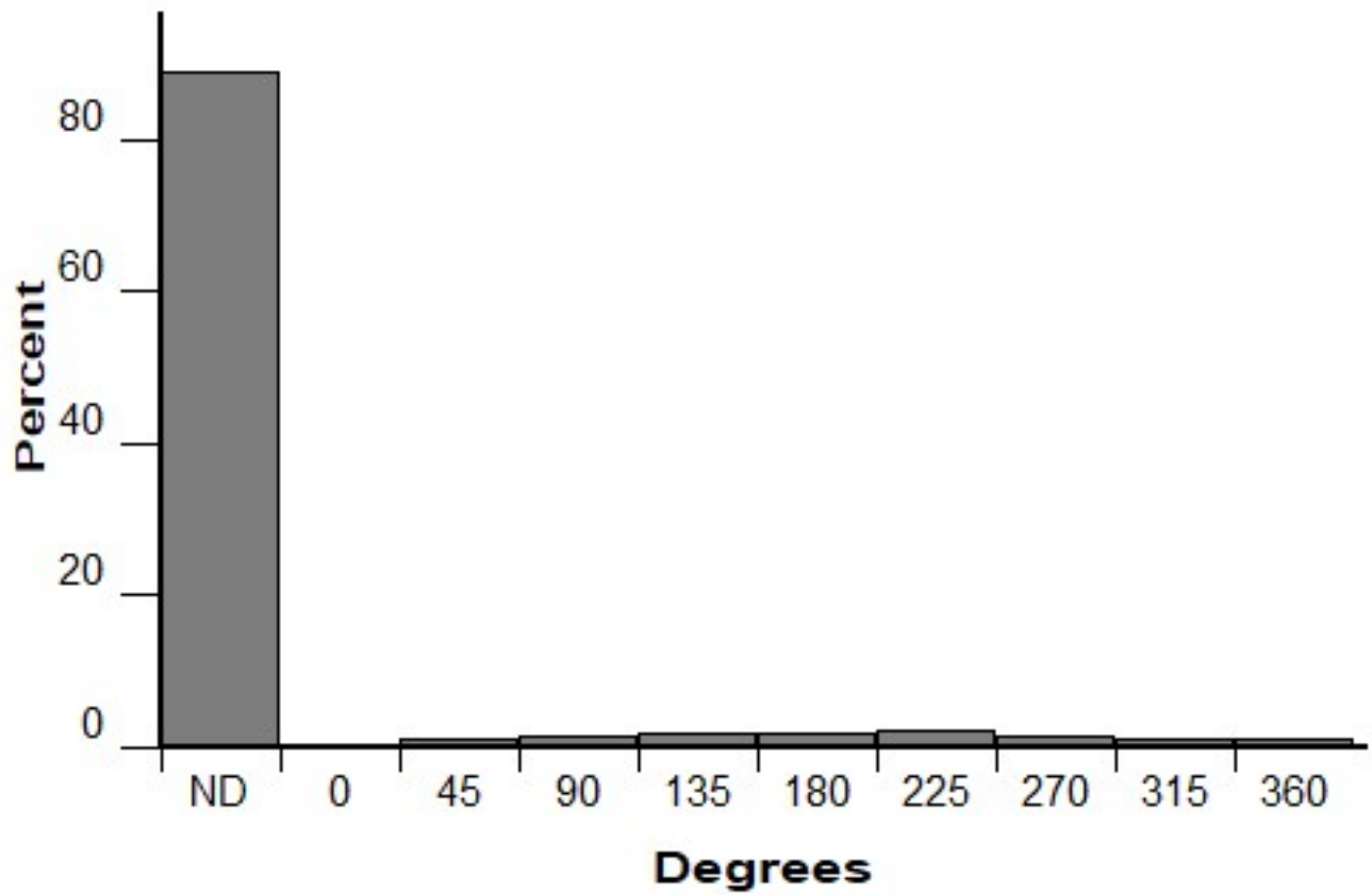
Aspect (FM 122)
