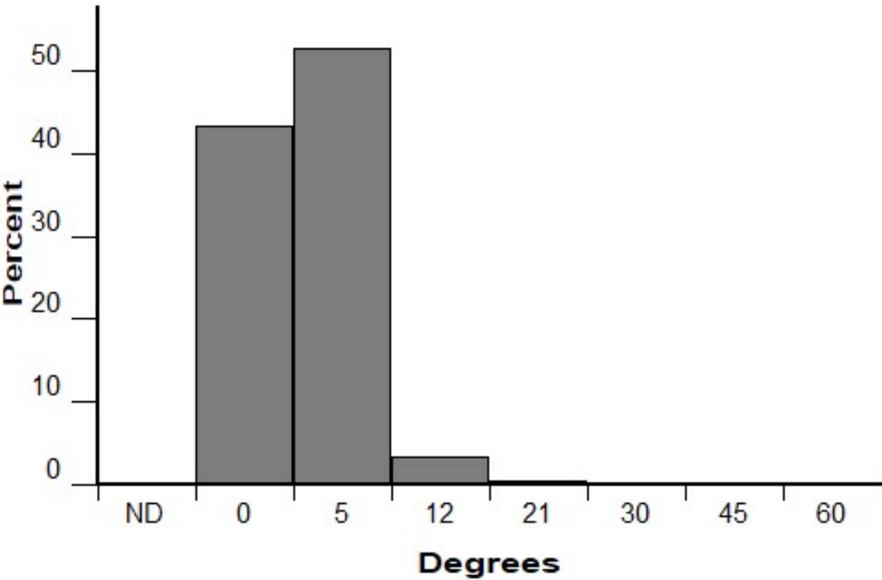
Slope (FM 122)
