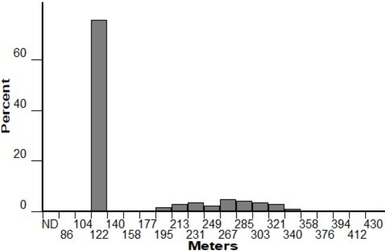
Elevation (FM 121)
