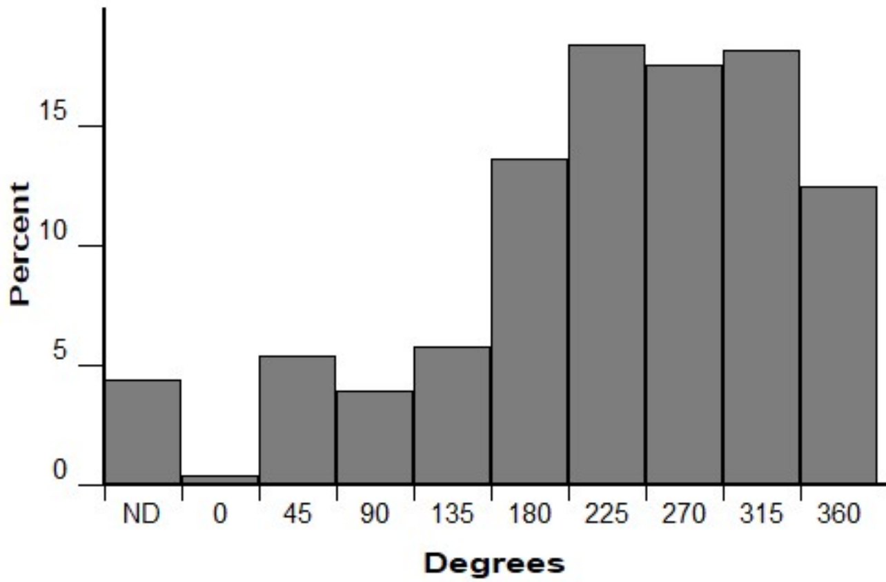
Aspect (FM 201)
