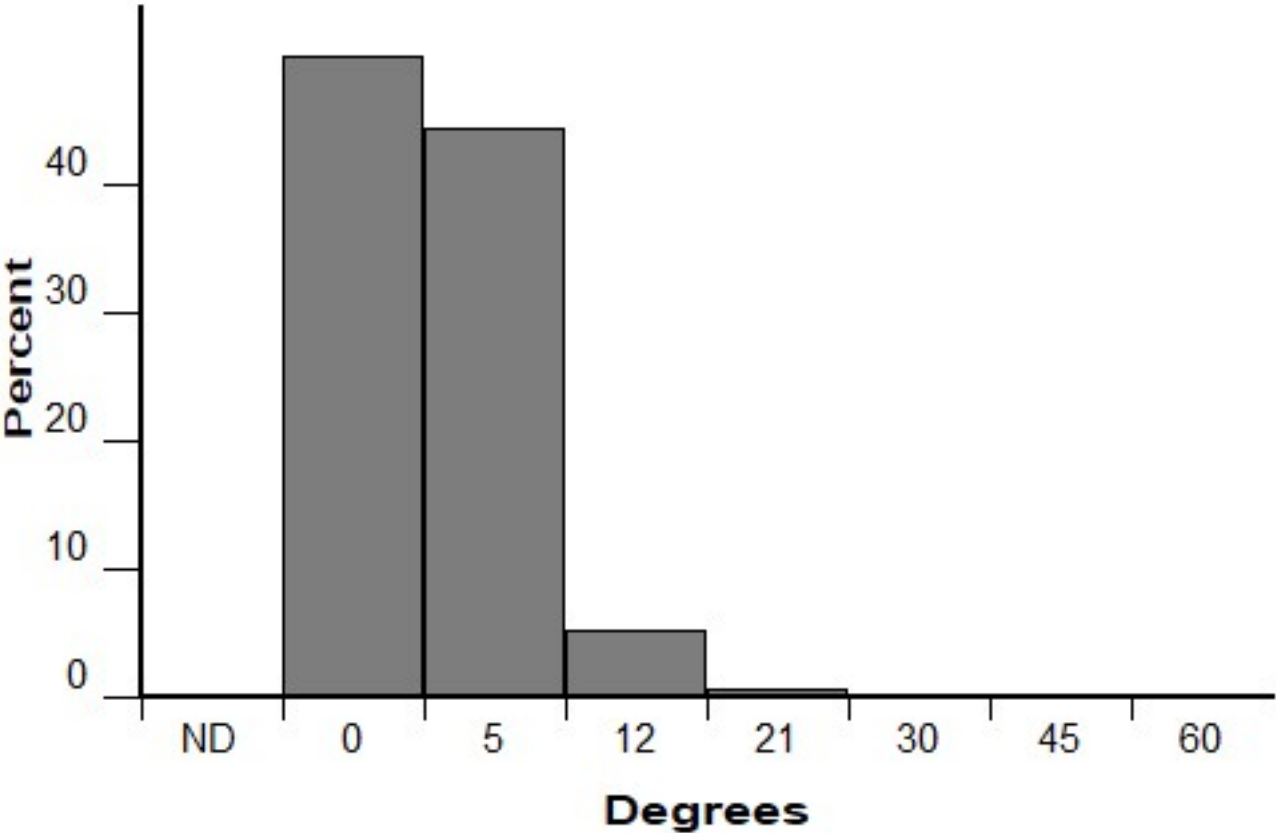
Slope (FM 98)
