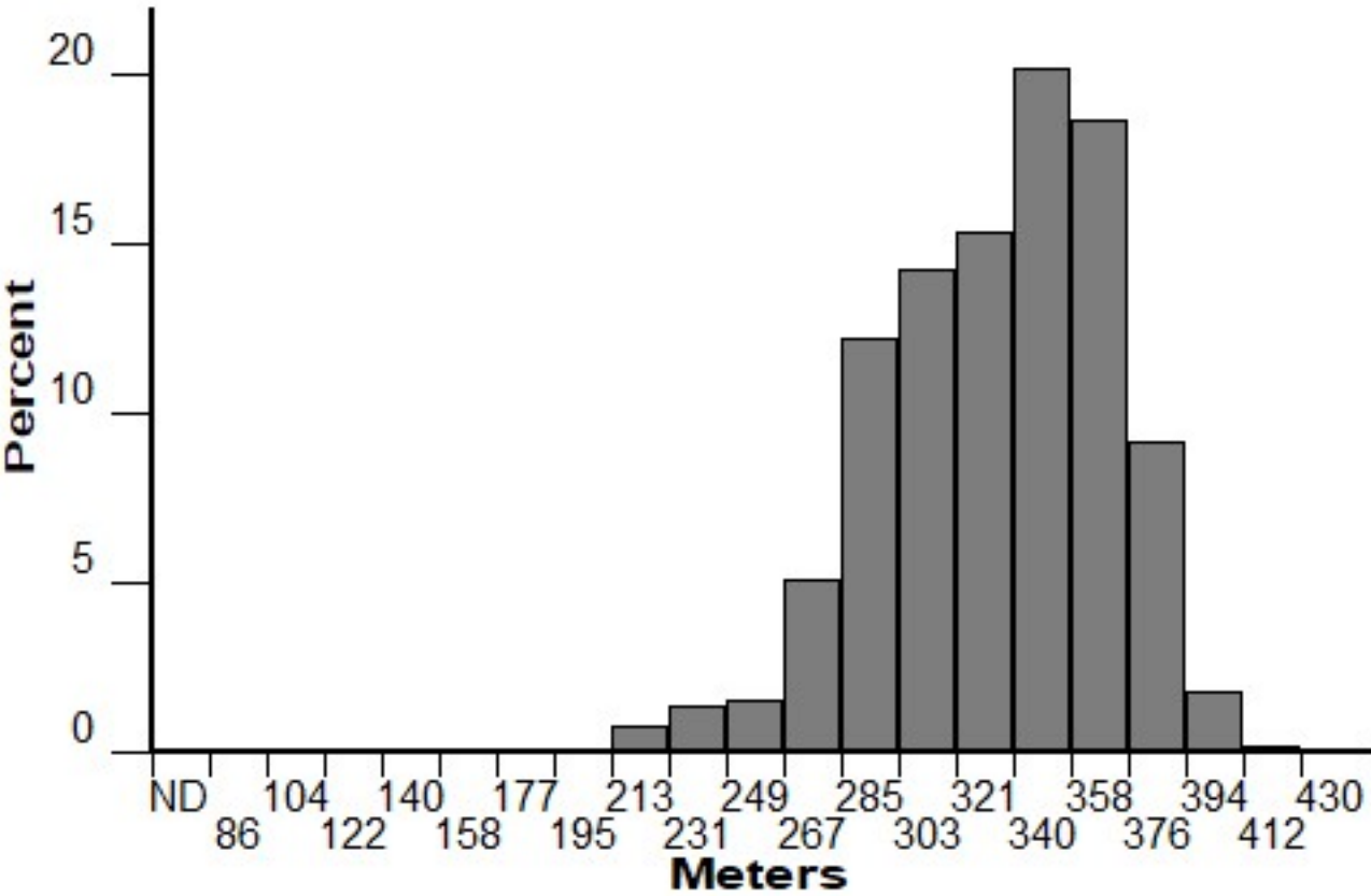
Elevation (FM 184)
