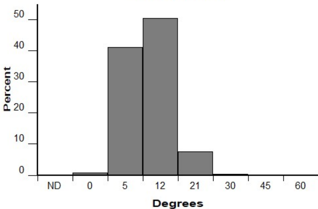
Slope (FM 186)
