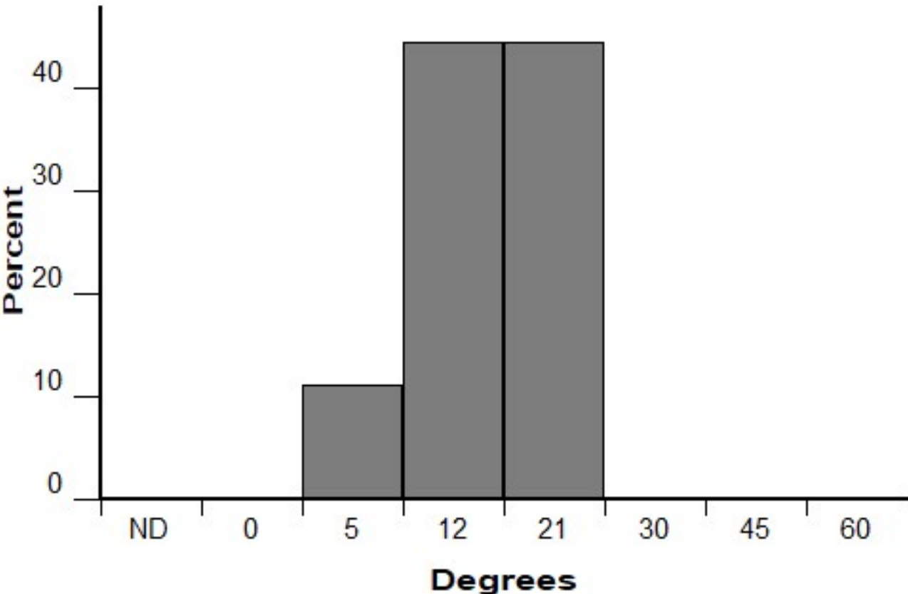
Slope (FM 202)
