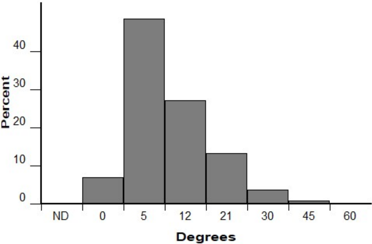
Slope (FM 99)
