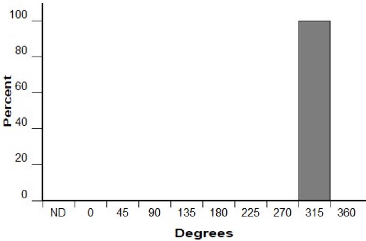
Aspect (FM 106)
