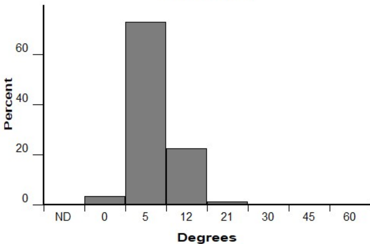
Slope (FM 91)
