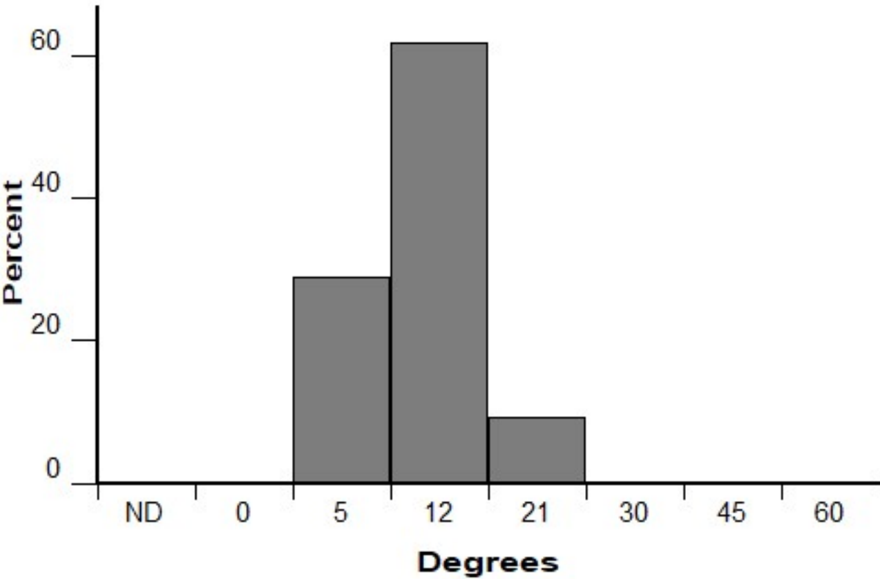
Slope (FM 162)
