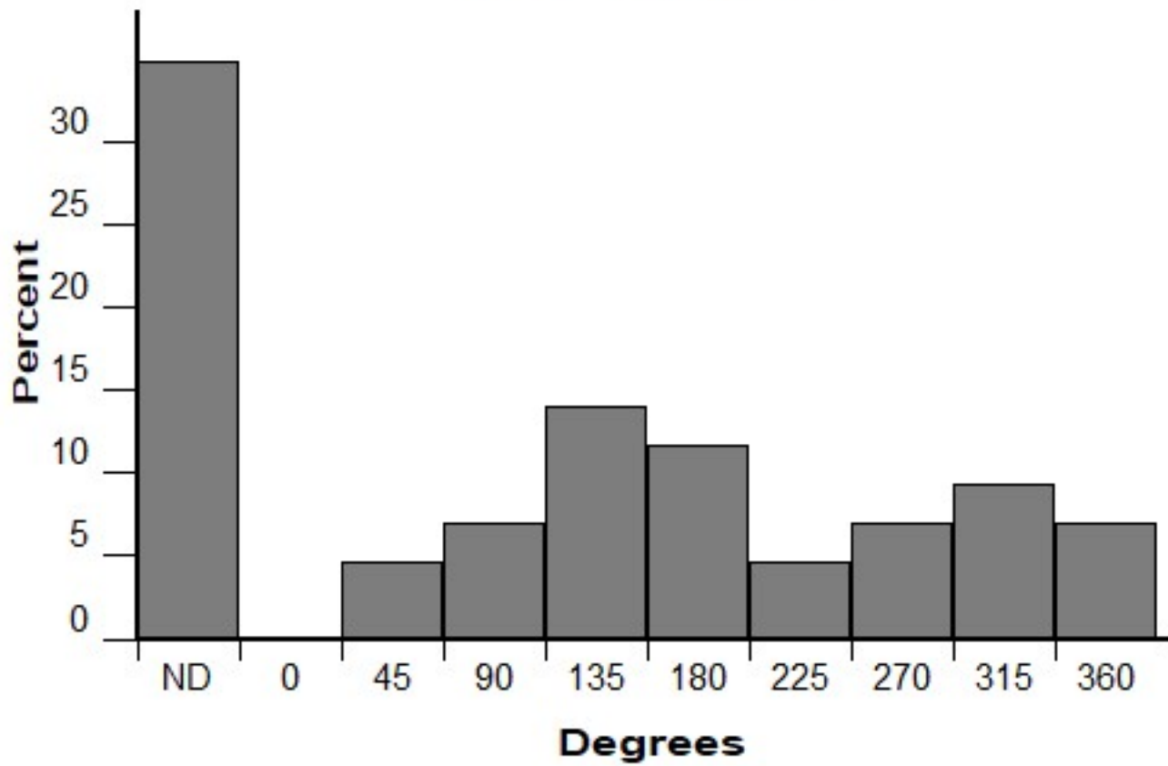
Aspect (FM 146)
