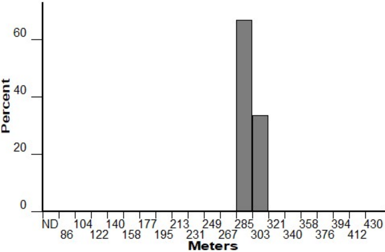
Elevation (FM 202)
