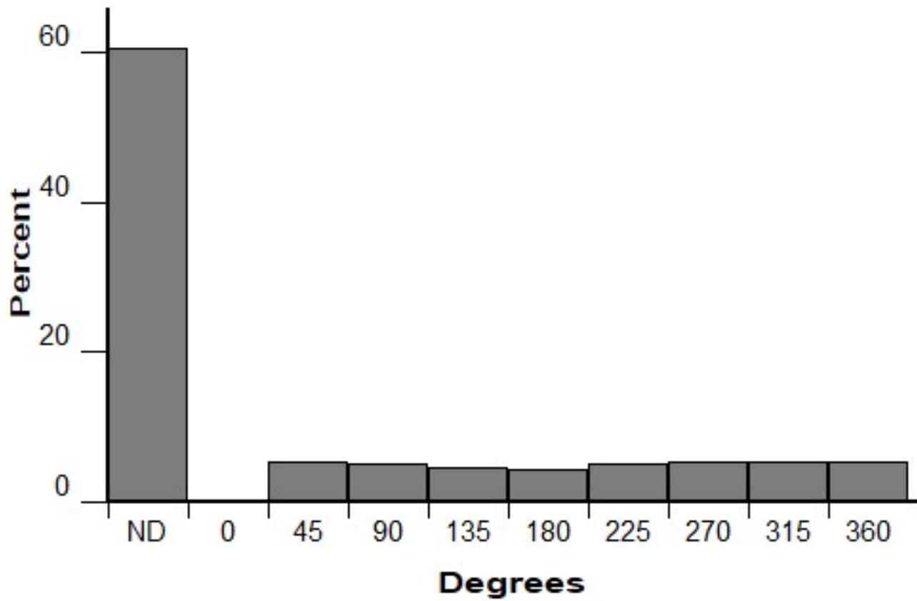
Aspect (FM 182)
