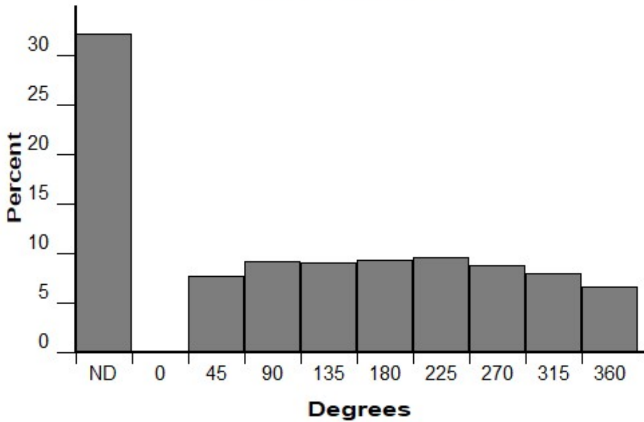
Aspect (FM 91)
