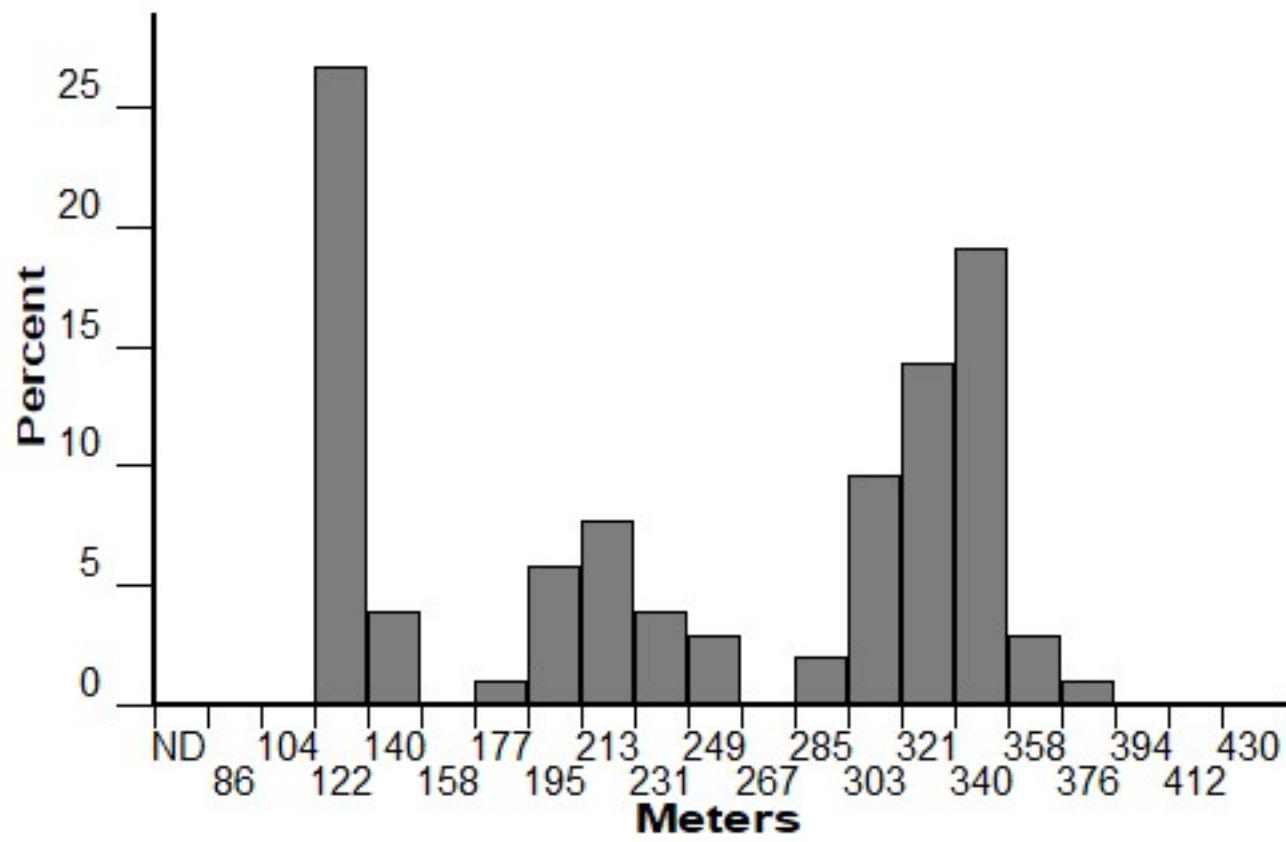
Elevation (FM 143)
