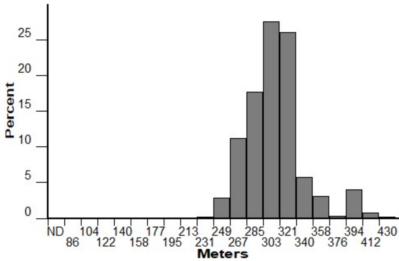
Elevation (FM 144)
