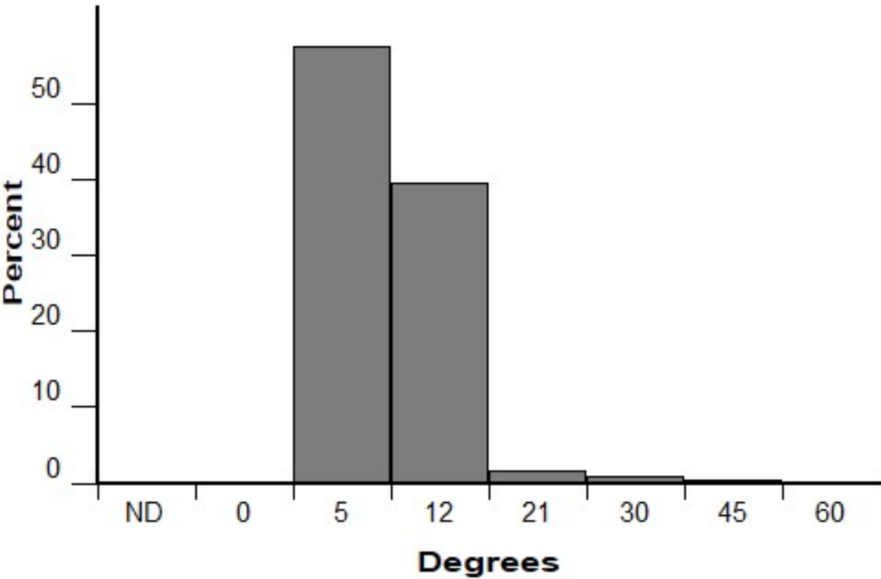
Slope (FM 142)
