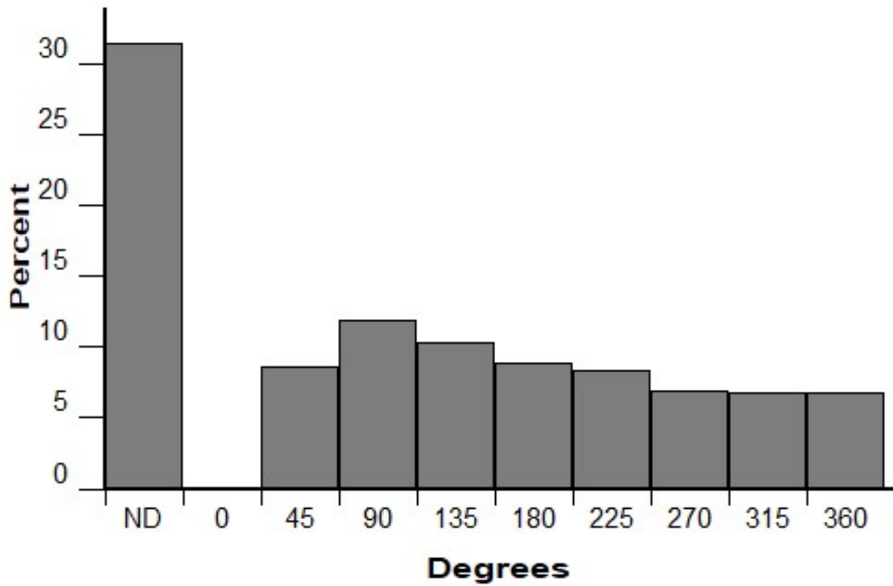
Aspect (FM 99)
