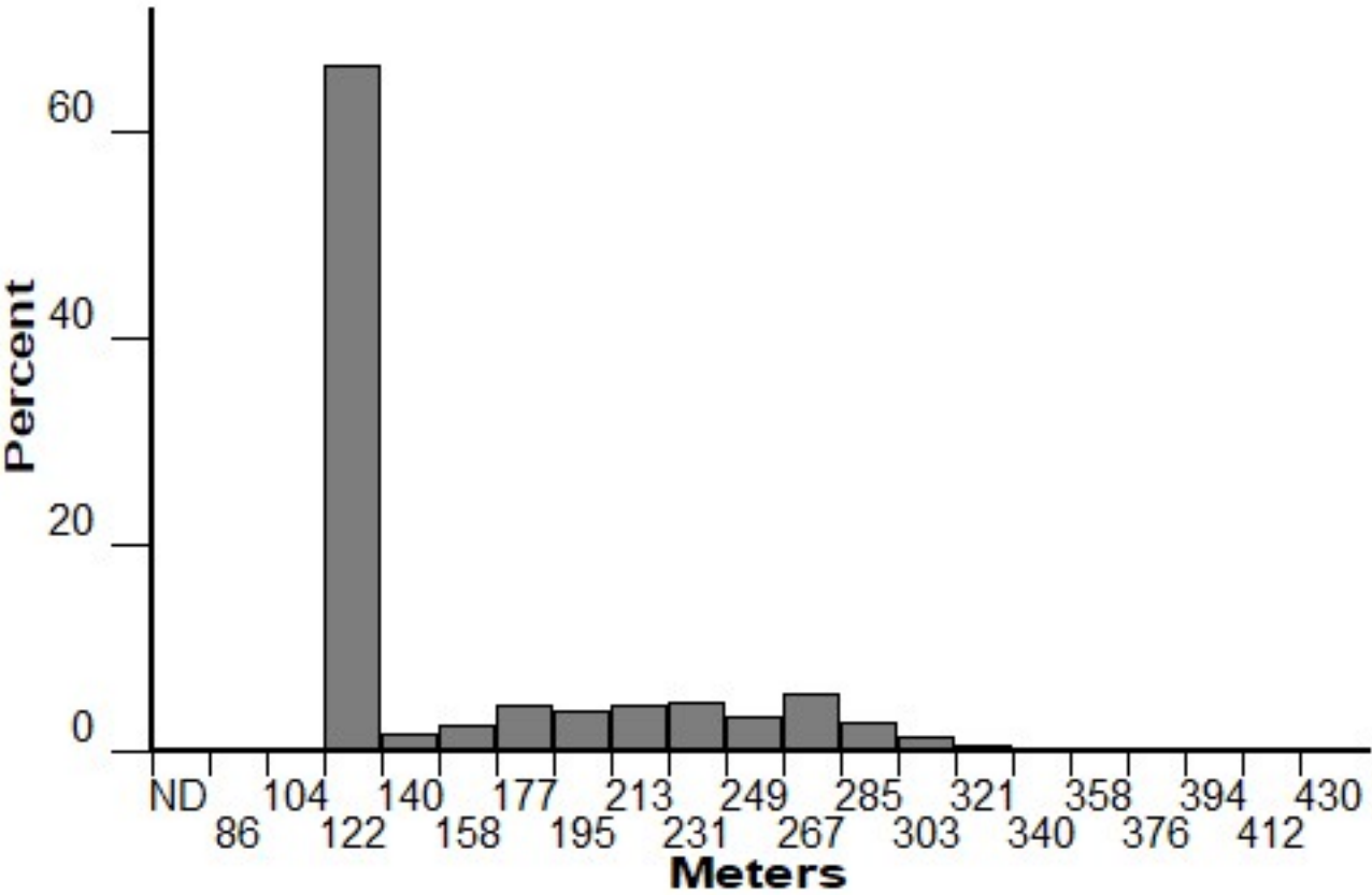
Elevation (FM 98)
