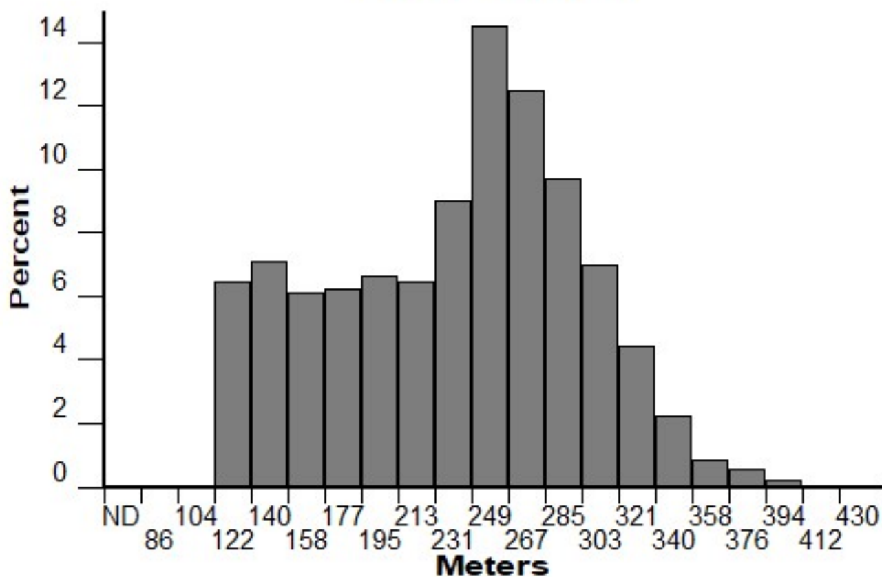
Elevation (FM 91)
