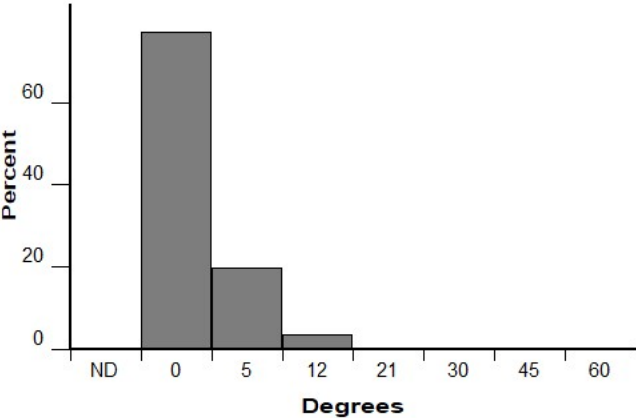
Slope (FM 121)
