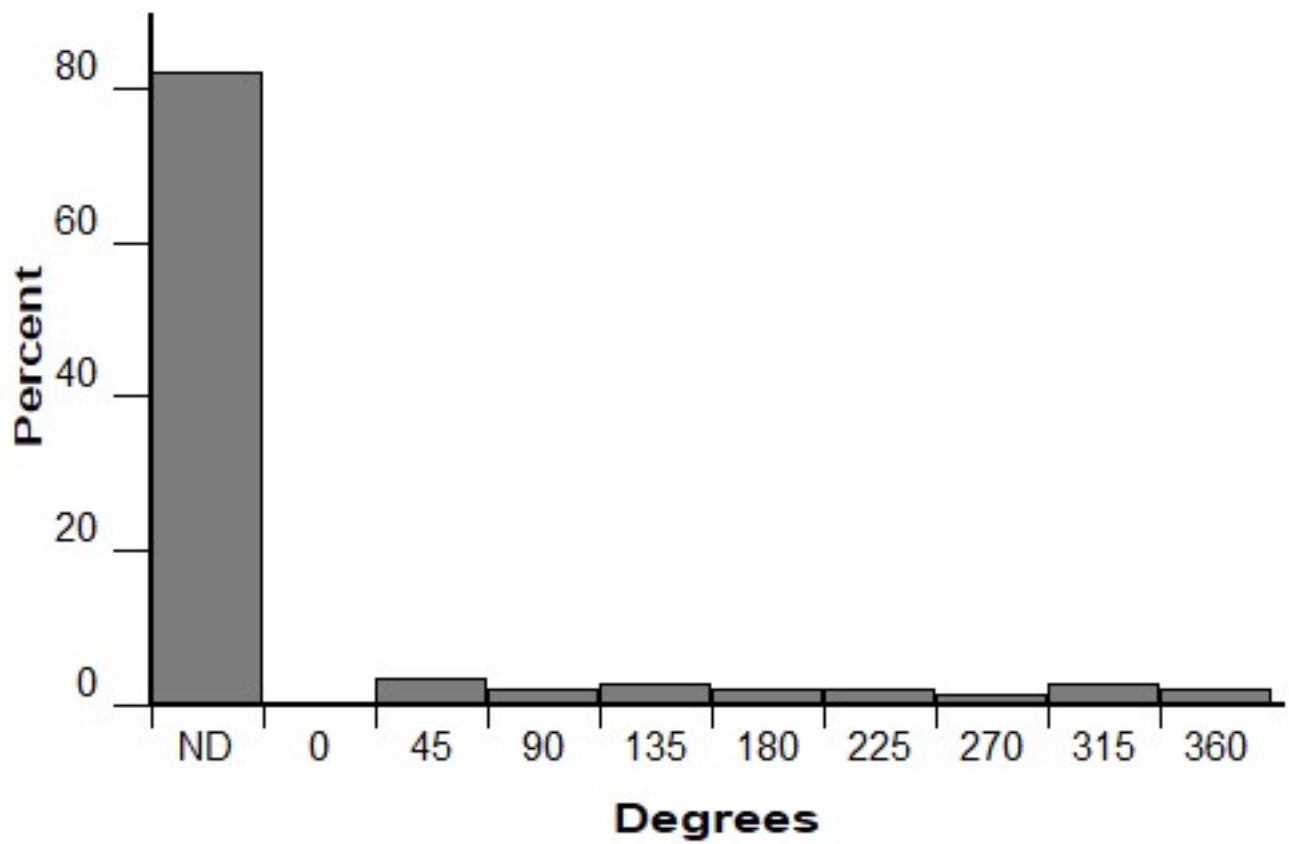
Aspect (FM 121)
