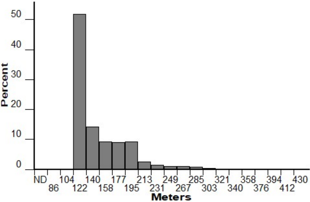
Elevation (FM 93)
