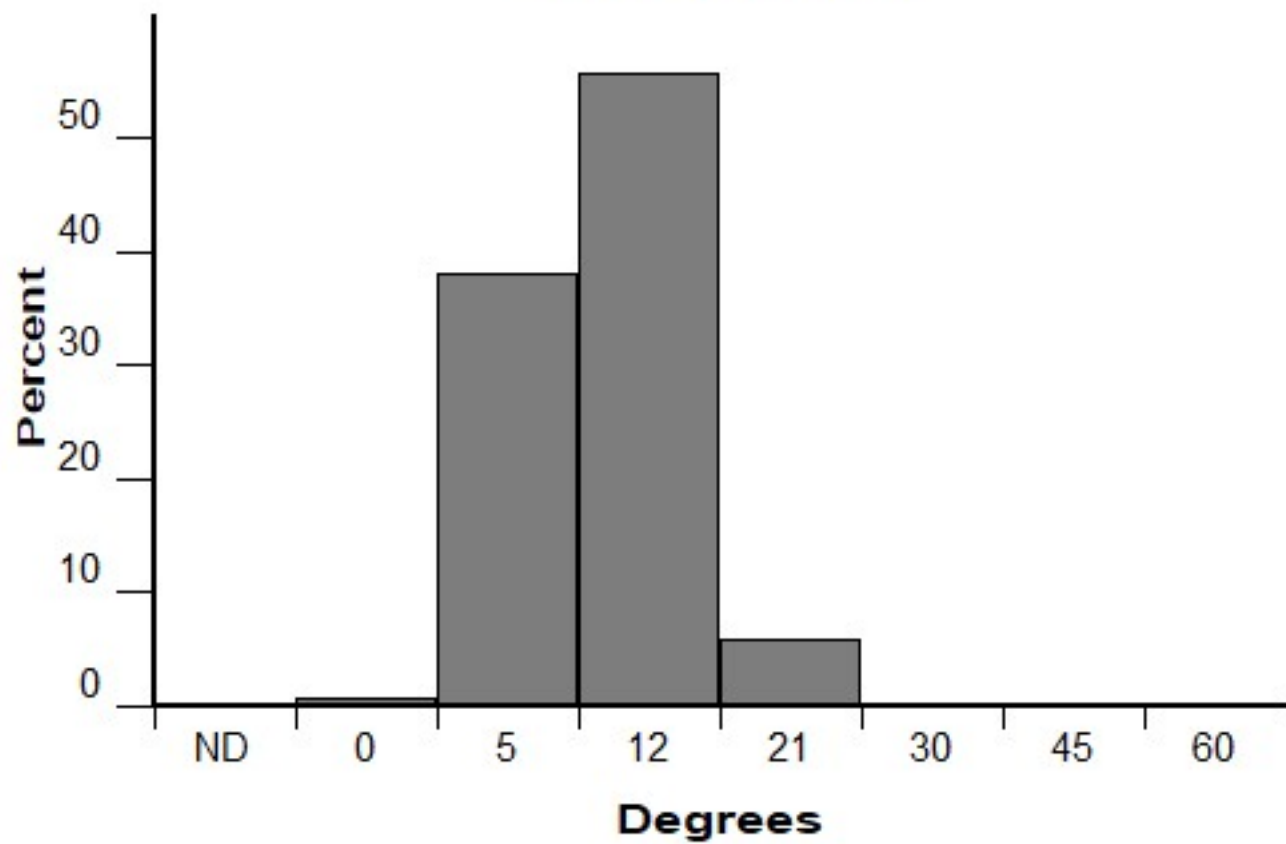
Slope (FM 181)
