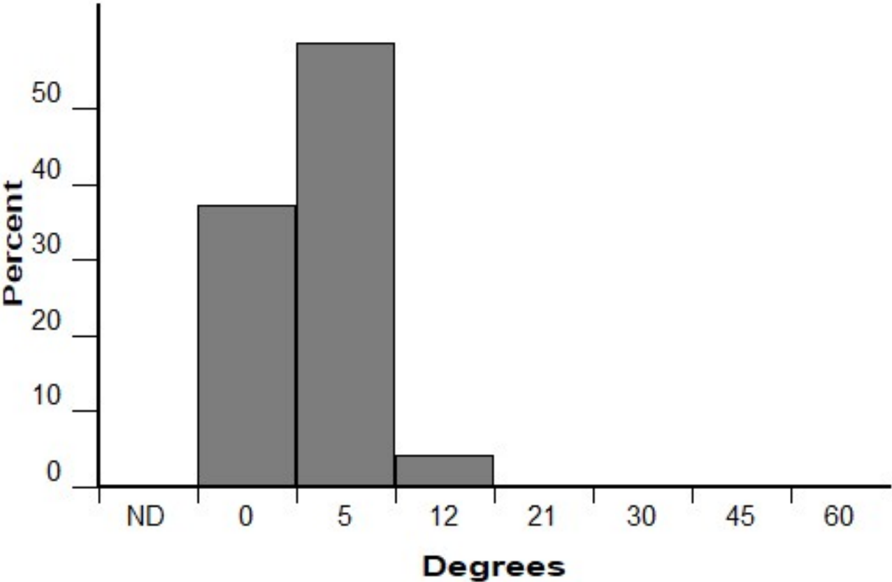
Slope (FM 93)
