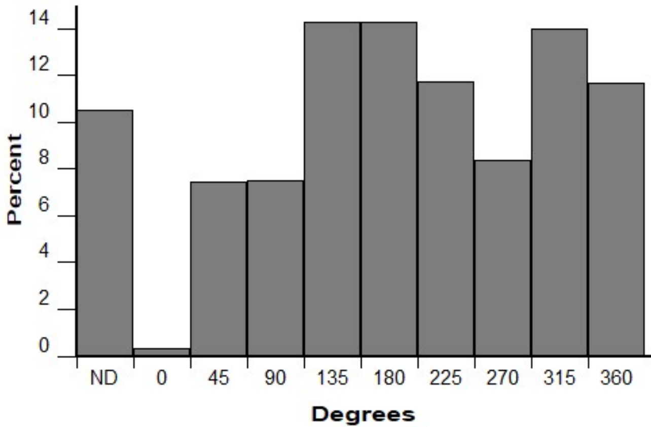
Aspect (FM 181)
