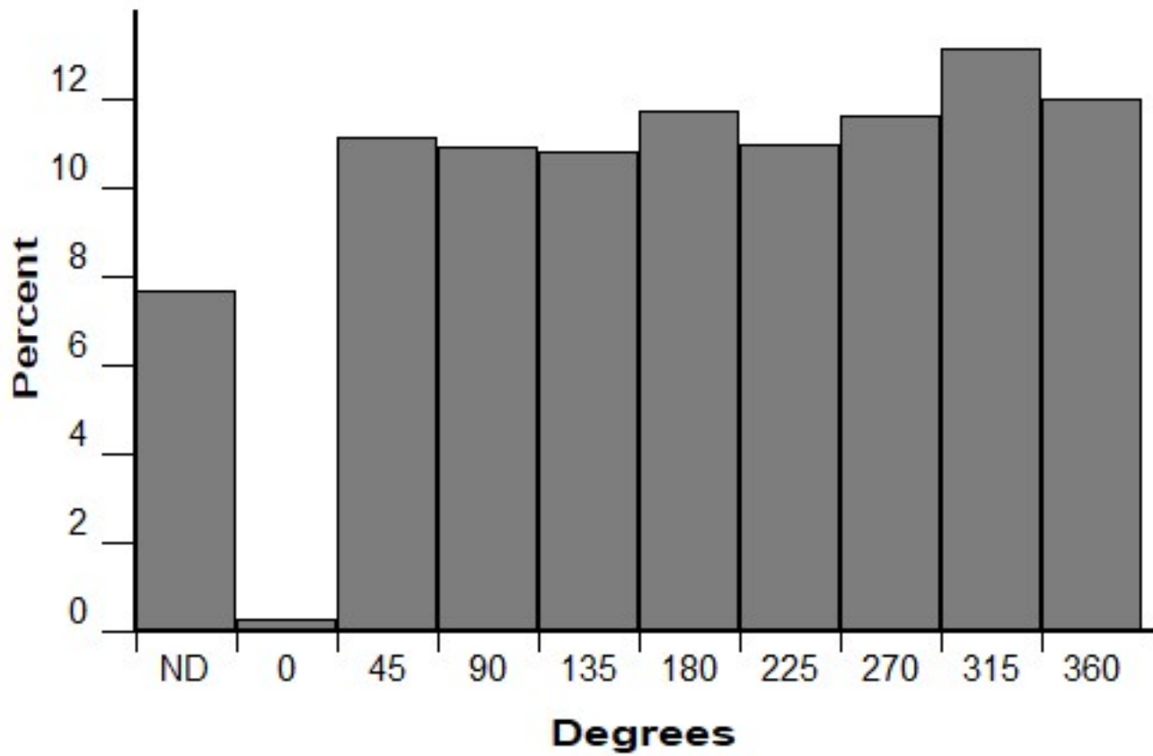
Aspect (FM 189)
